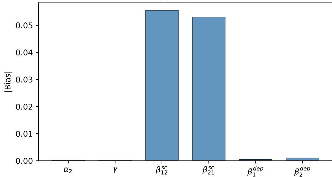
|Bias| per parameter
